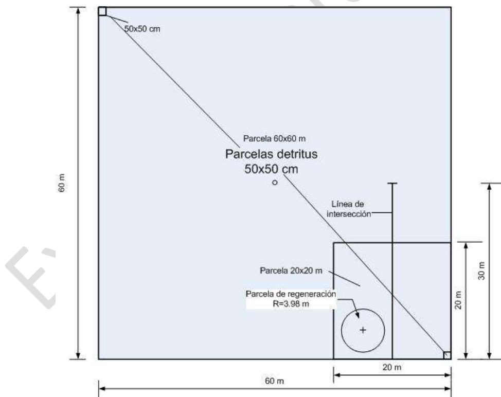
Figura 3. Diseño, distribución y tamaños de las parcelas anidadas donde se realizaron las diferentes mediciones.
