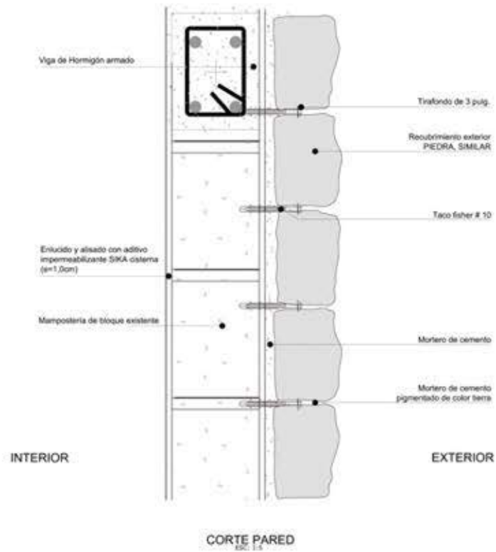
Gráfico 8: RECUBRIMIENTO DE PAREDES DE BLOQUE, PIEDRA
