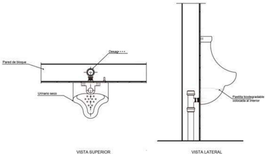
Gráfico 15: DETALLE DE URINARIO INSTALACIONES
