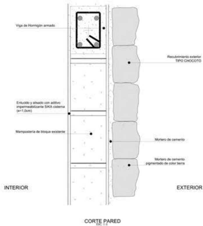
Gráfico 9: RECUBRIMIENTO DE PAREDES DE BLOQUE, CHOCOTO
