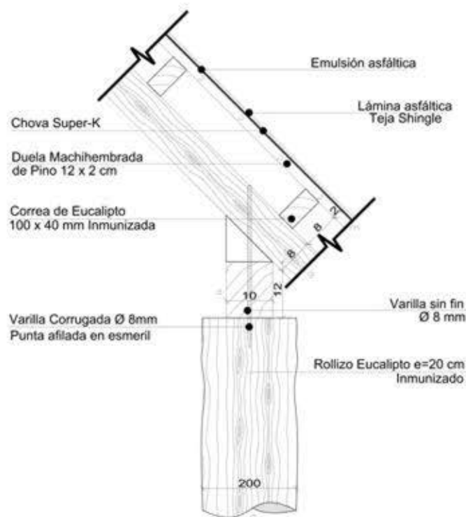
Gráfico 2: ARMADO CUBIERTA
