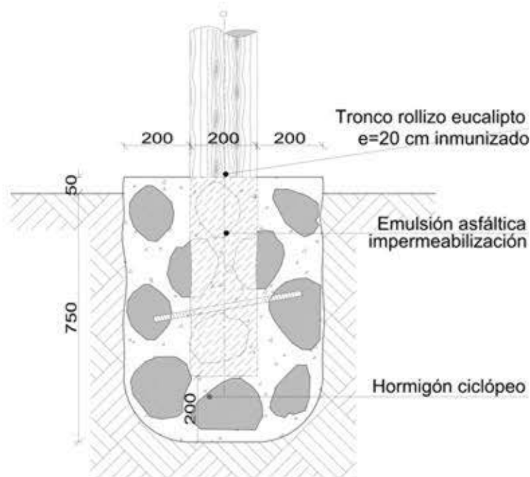
Gráfico13: CIMENTACION
