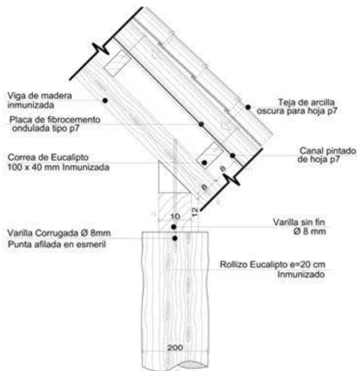
Gráfico 3: ARMADO CUBIERTA
